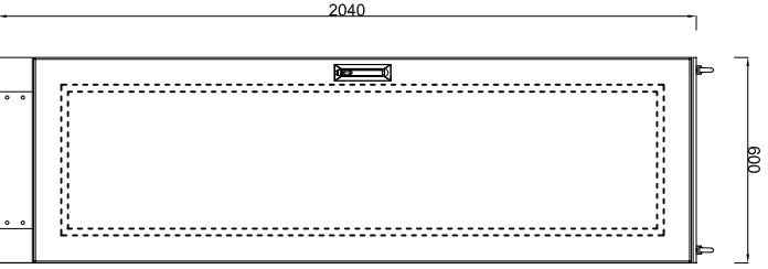
ÜST GÖRÜNÜM
