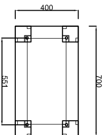
ALT GÖRÜNÜM
