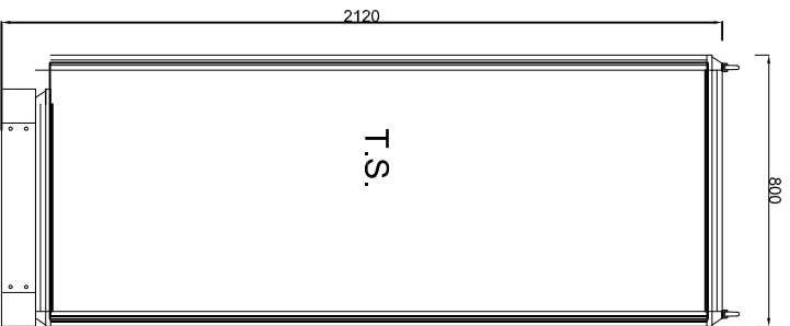
İÇ GÖRÜNÜM
