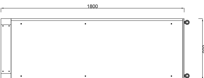
YAN GÖRÜNÜM
