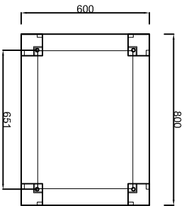
ALT GÖRÜNÜM
