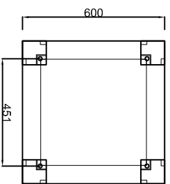
ALT GÖRÜNÜM
